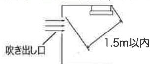
取付例
