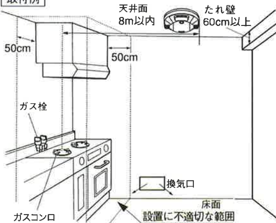
取付例
