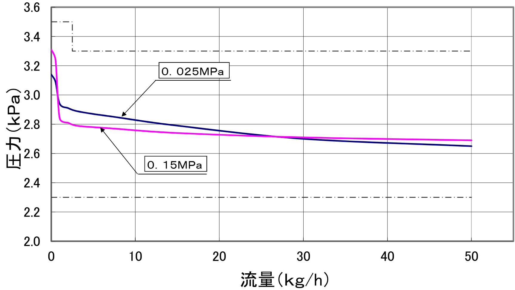
RL-50HL-II 性能曲線
