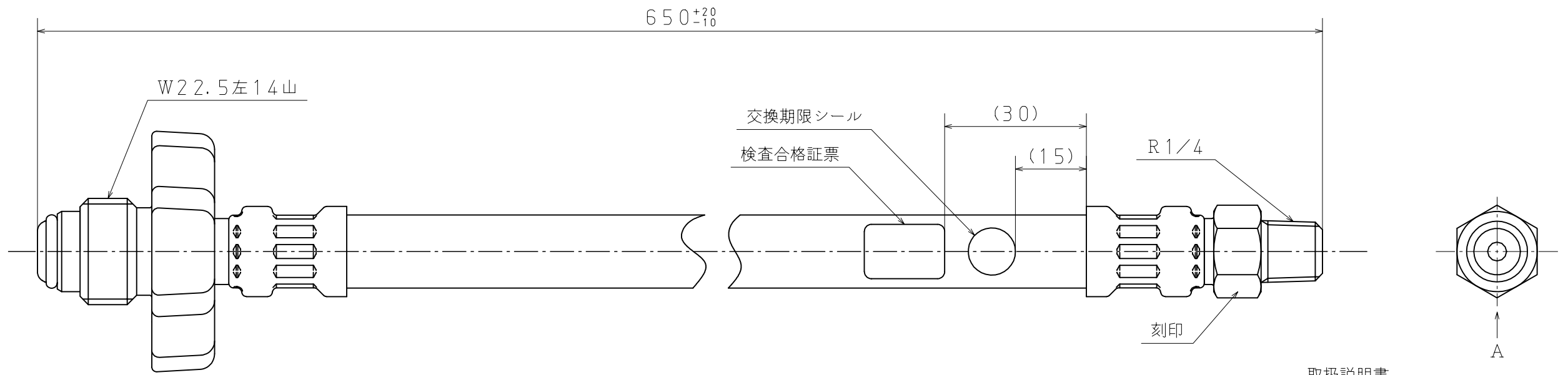
刻印の内容 (A矢視)
