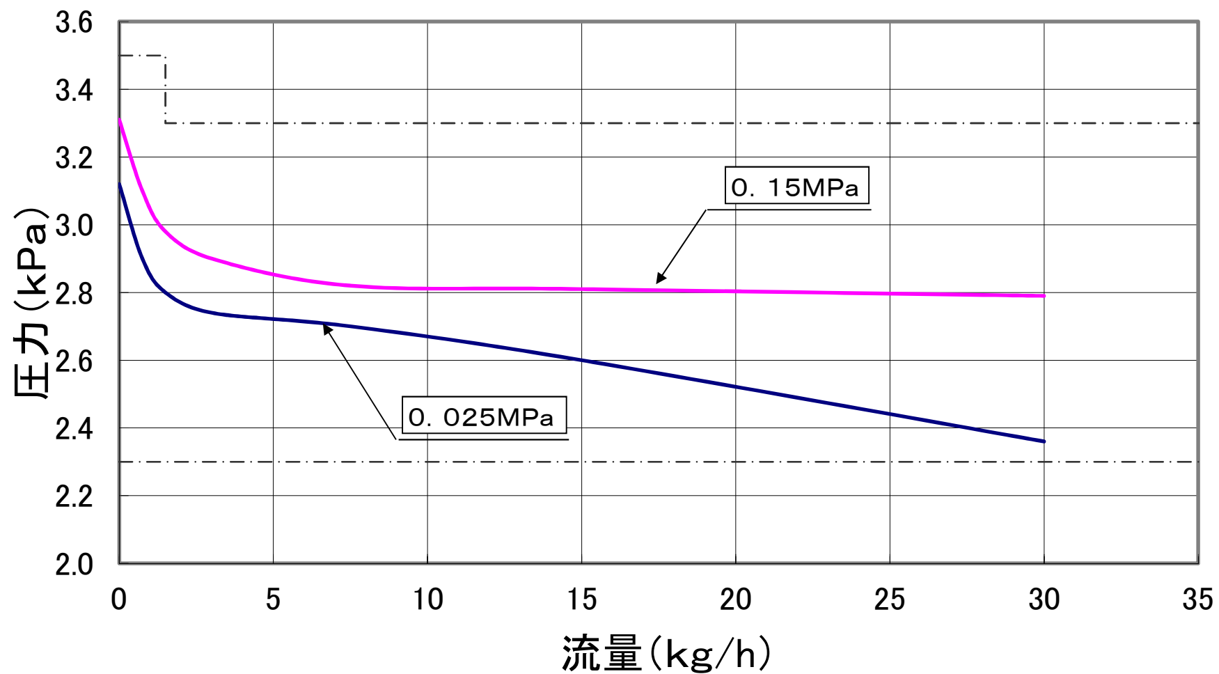
RL-30HL-II 性能曲線
